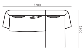
尺寸: 3200*1800*755mm 编码: 31F006ZH-01
